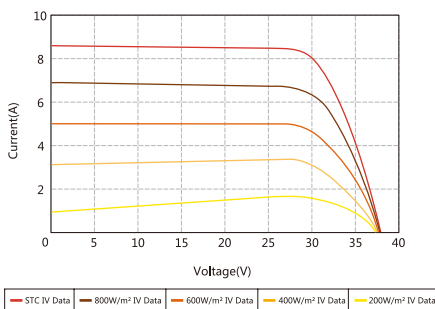
(AD250Q6-Ab) 出力特性図
