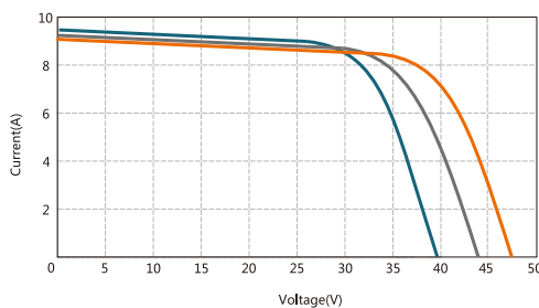
UL320P-72 電流・電圧(温度)曲線
