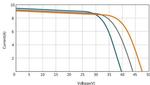
UL330M-72 電流・電圧(温度)曲線
